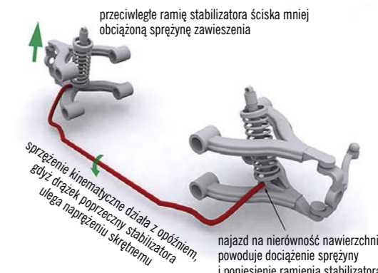
RYS. 18. DZIAŁANIE STABILIZATORA OGRANICZAJĄCE PRZECHYLEY NA ZAKRĘTACH
